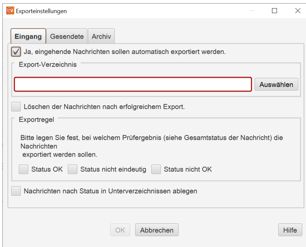
Abbildung 26: Exporteinstellungen, Register "Eingang"
